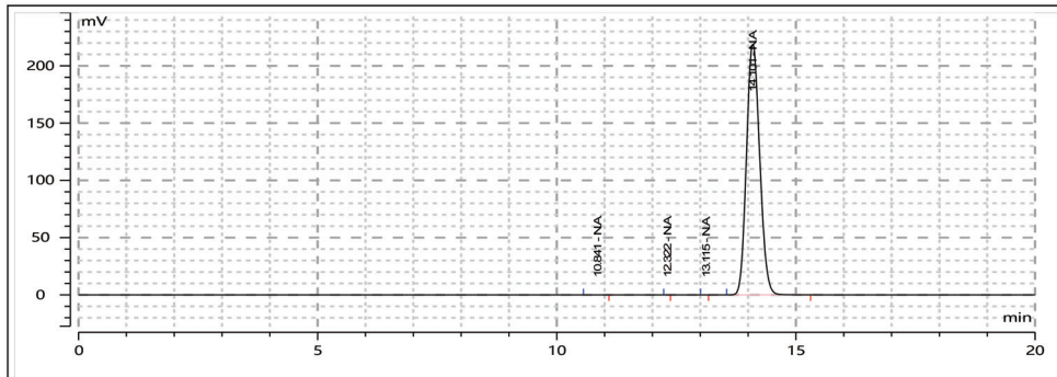
L-岩藻糖 -(BOX-通道1)
